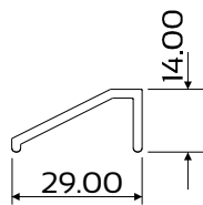
DIE No. W10083 Cas34 Add On Weather Bar
