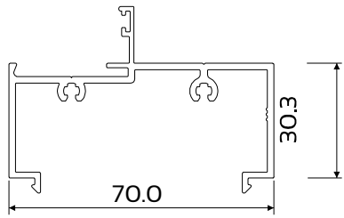
DIE No. W33135 Cas34 Frame 70mm
