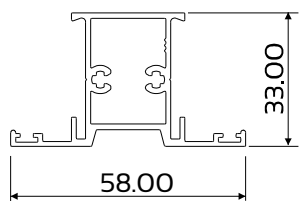
DIE No. W55692 Cas34 Mullion
