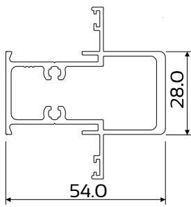
DIE No. W56269 Cas34 54mm Mullion
