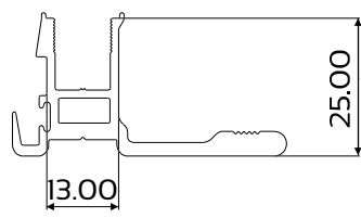
DIE No. W53888 Sash Interlocker
