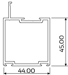
DIE No. W44093 Clip44 R3 Special Door Jamb
