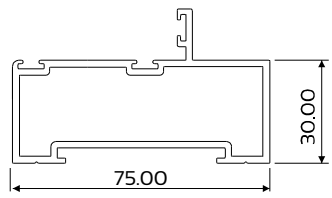
DIE No. W55111 Clip44 Jamb Vistafold
