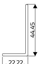
DIE No. W01405 44,45x22,22x2,03
