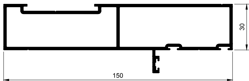
Horizon Jamb Rail W57566
